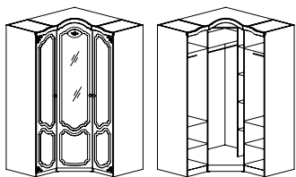
Шкаф для одежды СП-002-18 Д136 x В222 x Г136
