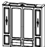
Шкаф для одежды МН-306-04 Д 207 см В 229 см Г 63 см
