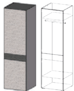
CO-1D szafa P, L W: 2062, S: 604, G: 571
