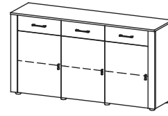
LU-K3 komoda W: 885, S: 1658, G: 440
