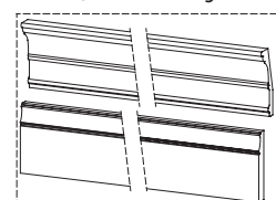
BA- cokół, korona do regałów bez boku zewnętrznego L, P (kpl.) W: 110, S: 426, G: 16 korona do regałów W: 110, S: 460, G: 50
