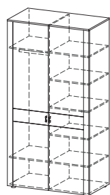
LU-2D szafa W: 2200, S: 1156, G: 600
